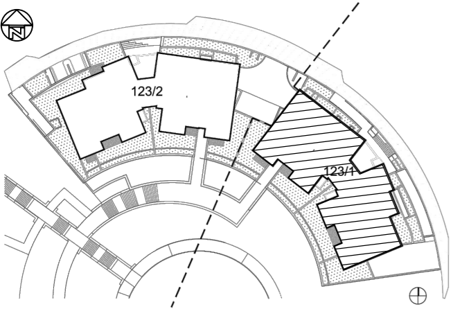
תכנית קומה: 1500
