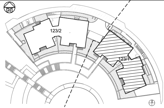
תכנית קומה 1500
